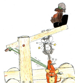
catapulta
